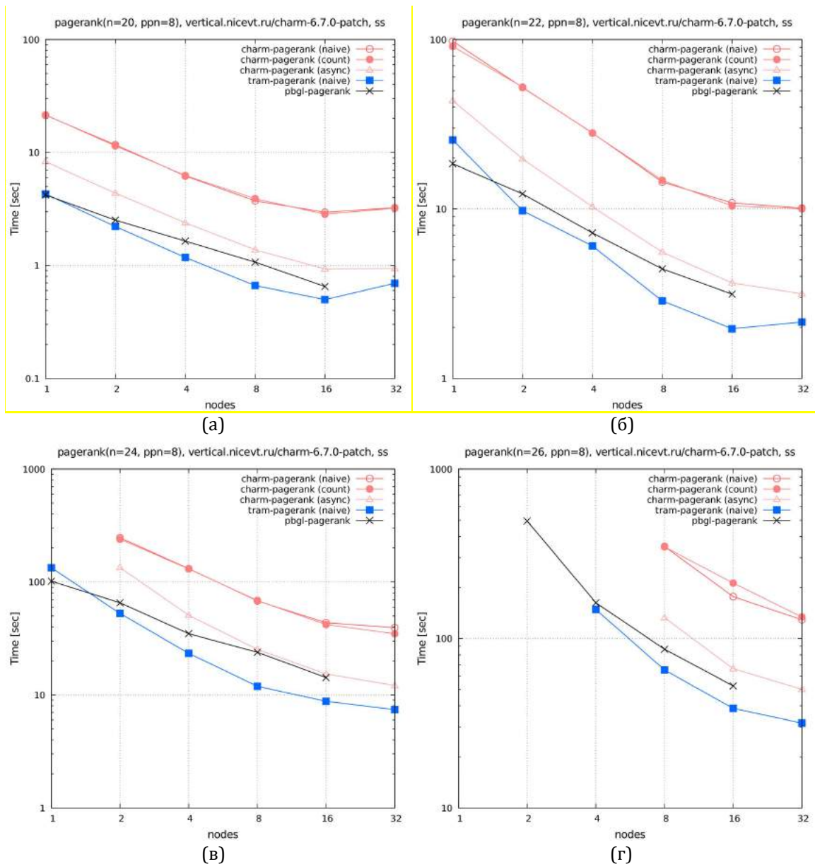
Рис. 5. Время выполнения PageRank на кластере Ангара-К1 для графов RMAТ-20 (а), RMAТ-22 (б), RMAТ-24 (в), RMAТ-26 (г). Режим сильной масштабируемости
